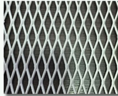
Chapa expandida espessura 2,00mm malha 11x42mm
