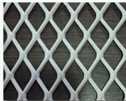
Chapa expandida espessura 1/8" (3,00mm) malha 20x50mm
